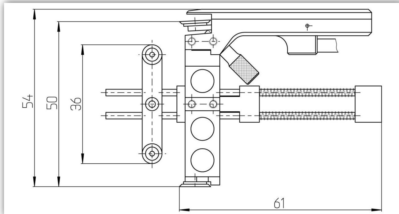
Bild 1: Mini MFA mit L_e 50
