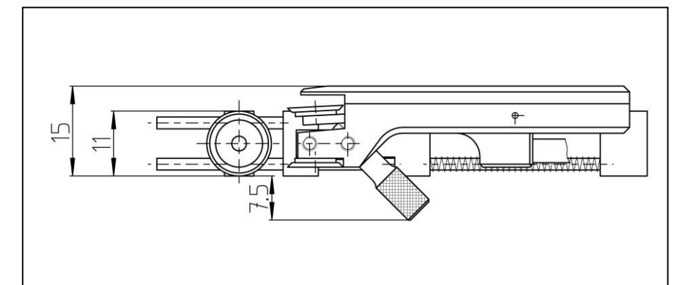
Bild 3: Mini MFA 2 mit L_e 10 und Sondergegenrolle \varnothing 10 mm
