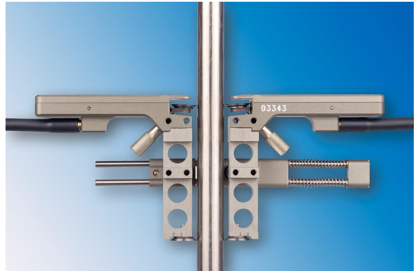
Bild 2: Mini MFA 2 doppelseitig
