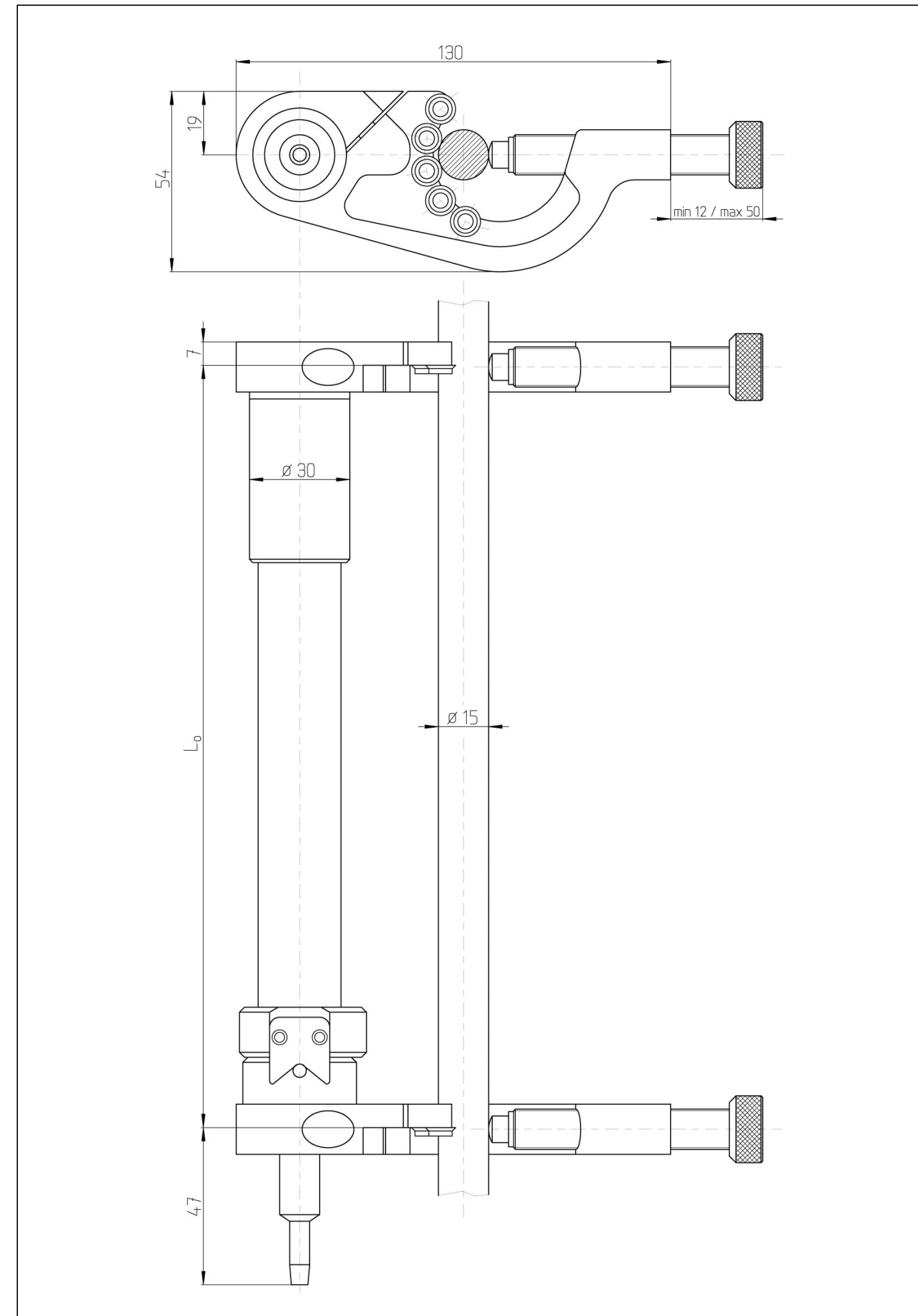
Bild 3: MFI - Abmessungen
