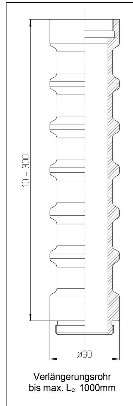
Bild 2: Verlängerungsrohr
